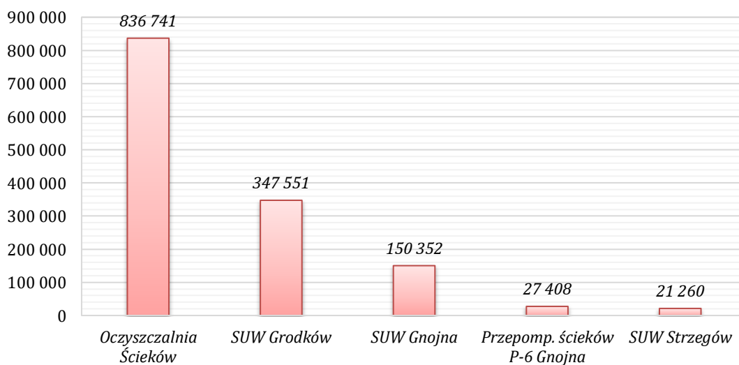
Wykres 57. Zużycie energii elektrycznej przez najbardziej energochłonne obiekty infrastruktury wod.-kan. na terenie Gminy Groduków [kWh]
